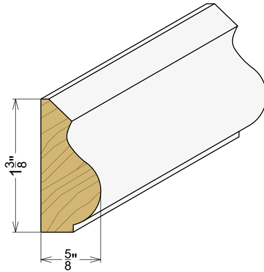
AP 1011 5/8" x 1-3/8"
