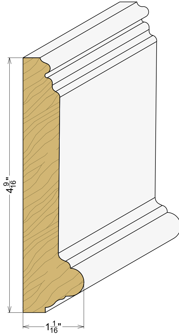
AP 2624 1-1/16" x 4-9/16"
