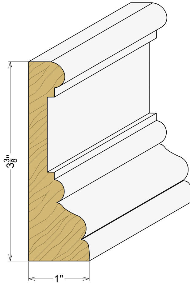
AP 2074 1" x 3-3/8"
