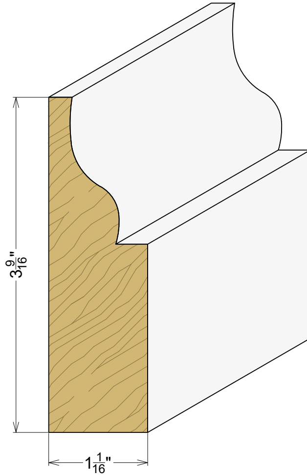
AP 2272 1-1/16" x 3-9/16"
