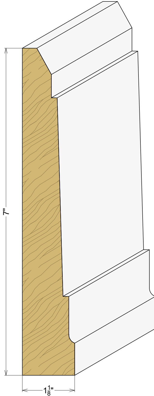
AP 4318 1-1/8" x 7"
