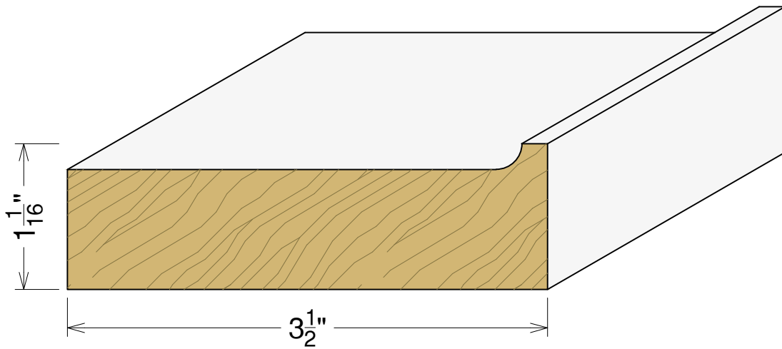
AP 5511 1 1/16"x 3 1/2"
