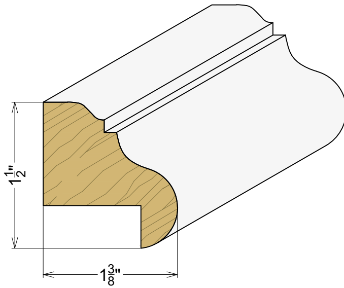
AP 6261 1-3/8" x 1-1/2"
