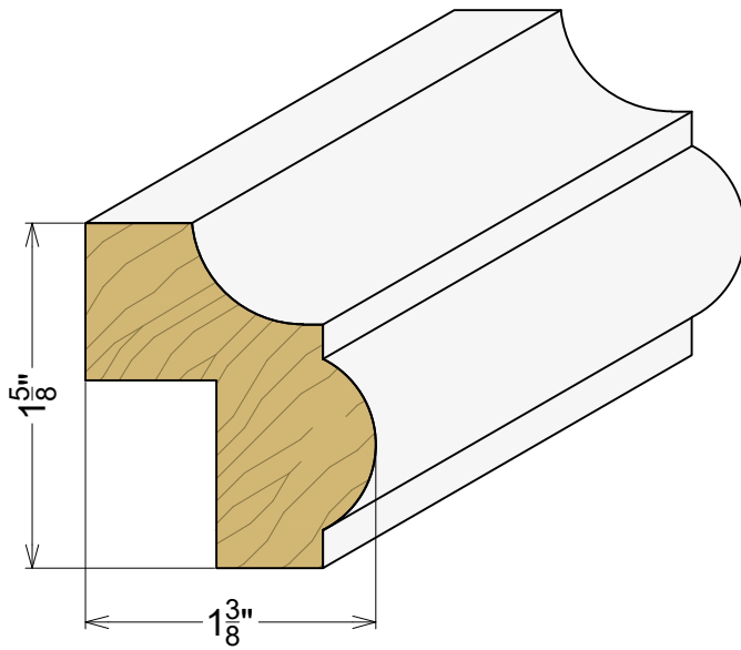
AP 6346 1-3/8" x 1-5/8"
